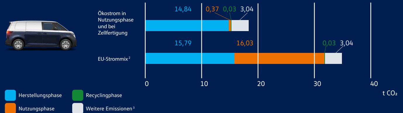
Vollständige CO 2 -Emissionen nach Lebenszyklusphase ohne Berücksichtigung von Kompensation: ID. Buzz Cargo 150 kW 82 kWh (brutto) (Modelljahr 2023) 1
